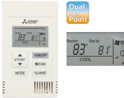
PAC-YT53CRAU (MA) Dimensions: 2-3/4(W) x 4-3/4(H) x 19/32(D) in. : 70(W) x 120(H) x 14.5(D) mm
